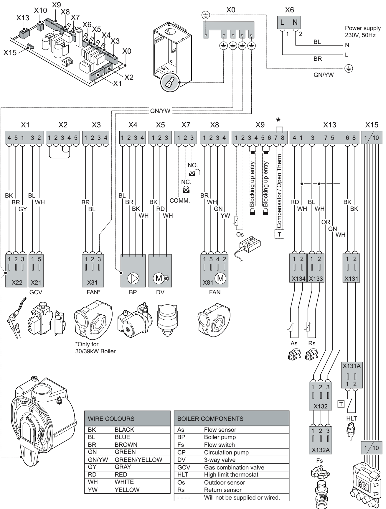
fig. 31 Diagrama del cableado LT.AL.W7H.000.234
