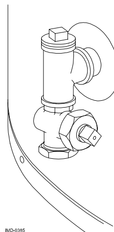
Dibujo 3: grifo de evacuación
