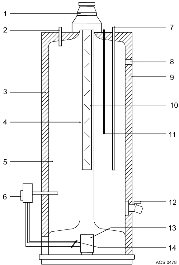
Imagen 1 - Corte transversal del calentador
