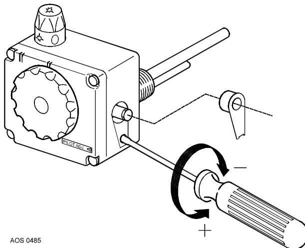
Imagen 8 - El ajuste de la llama piloto
