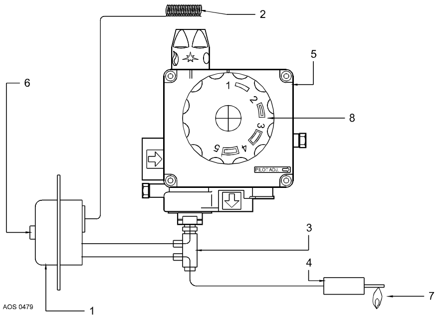
Imagen 2 - Bloque regulador para el suministro de gas con P.C.T.
