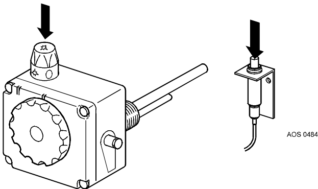
Imagen 6- Mando de la unidad reguladora para el suministro de gas
