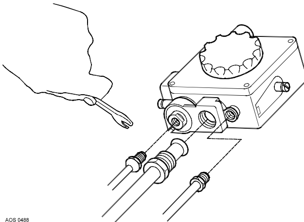
Imagen 11 - Montaje del juego del quemador
