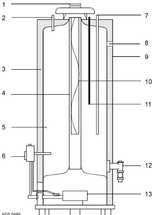
Imagen 1 - Corte transversal del calentador
