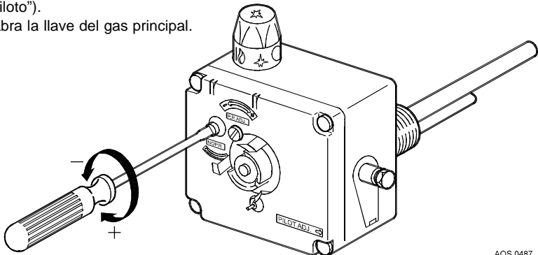
Imagen 9 - Cambio a otro tipo de gas
