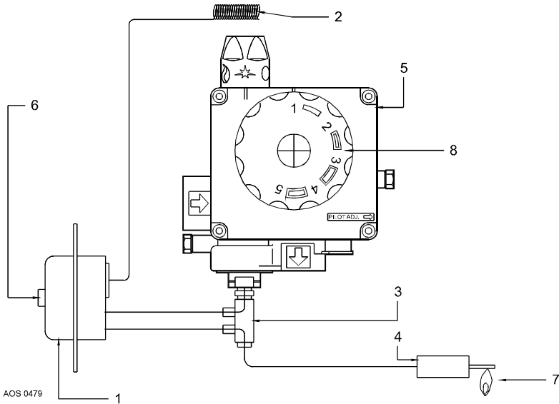
Imagen 2 - Bloque regulador para el suministro de gas con P.C.T.
