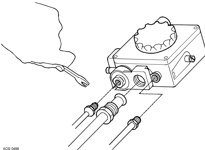
Imagen 10 - Montaje del juego del quemador
