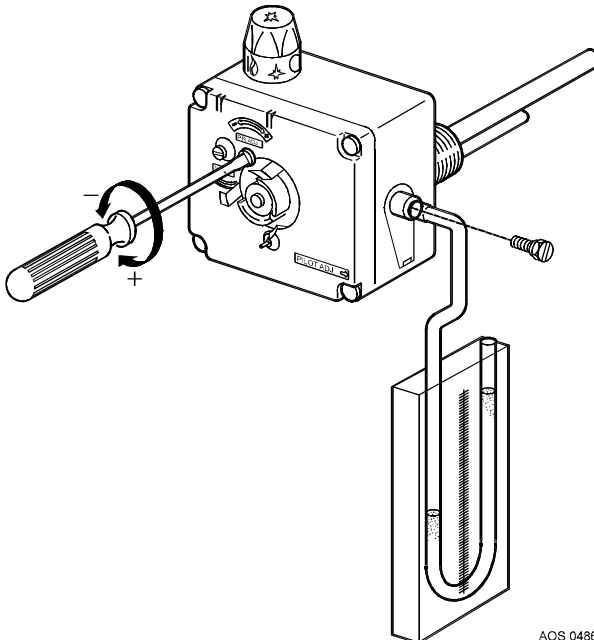
Imagen 8 - El ajuste de la carga nominal
