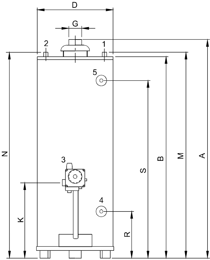
Imagen 3 - Medidas
