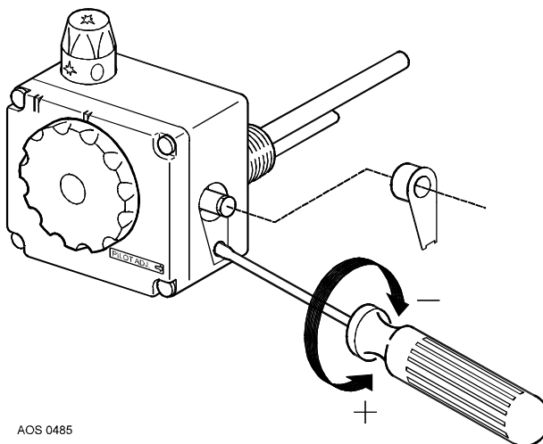
Imagen 7 - El ajuste de la llama piloto
