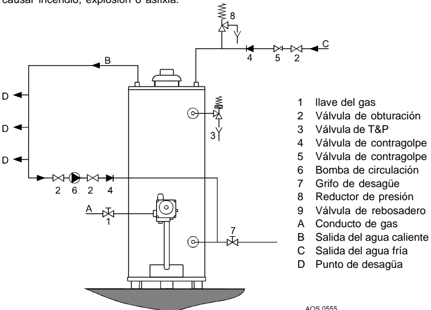
Imagen 4 - Esquema de la conexión
